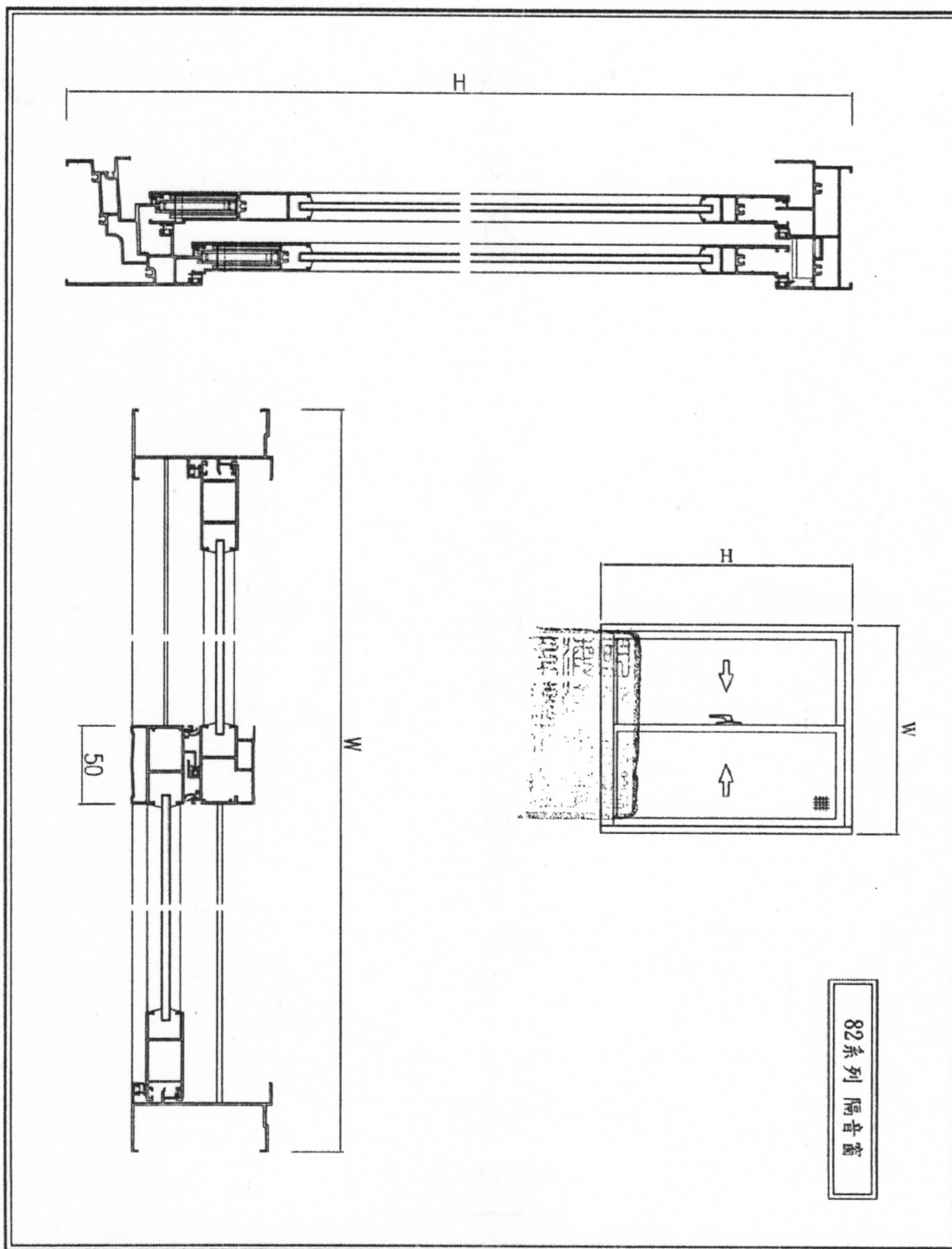
圖 3 試樣結構圖
